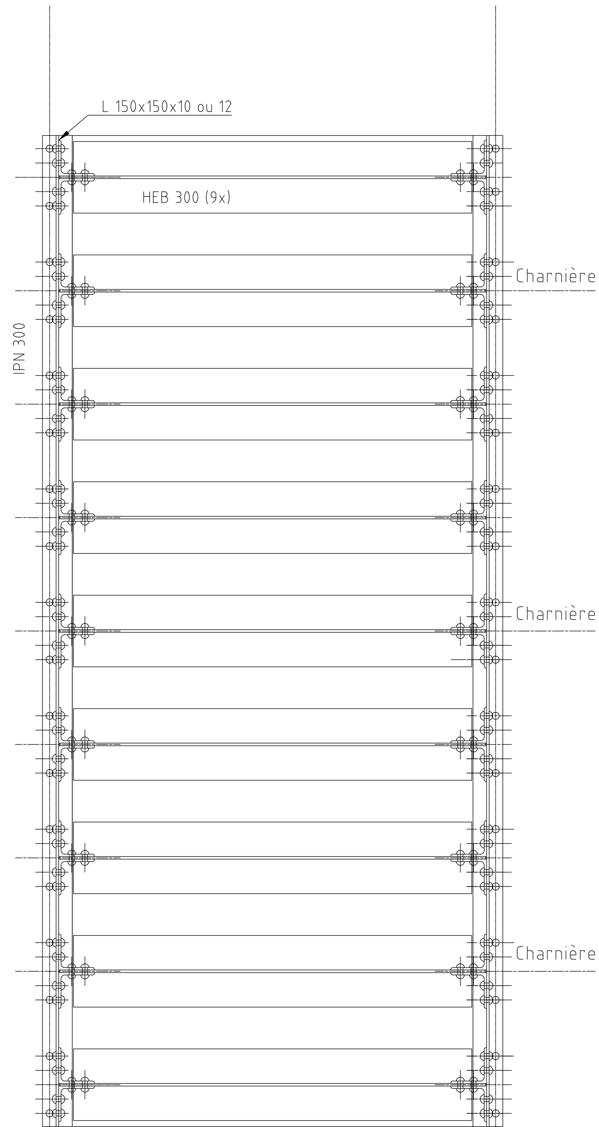
Coupe verticale dans le plan
