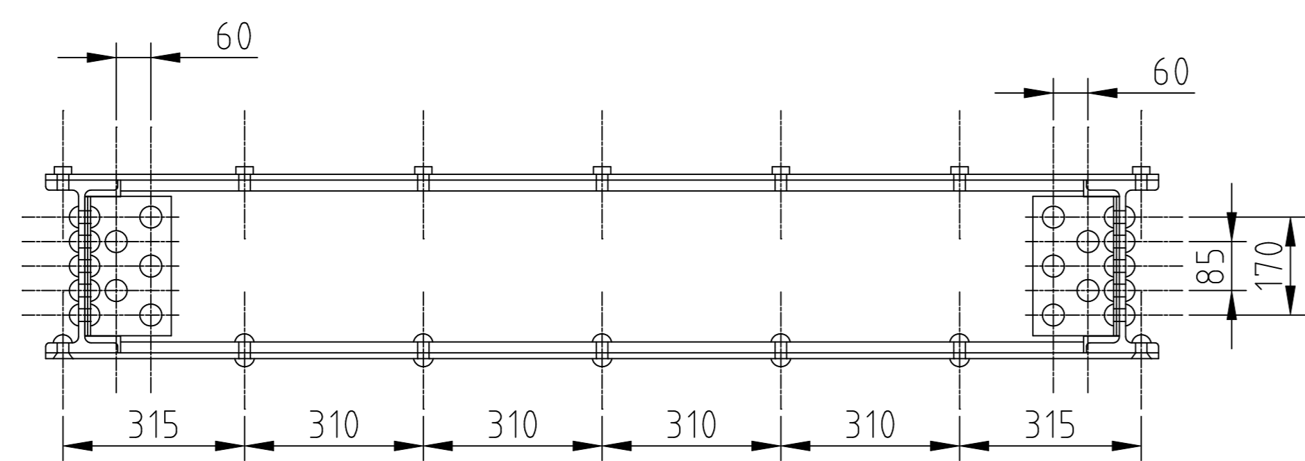
Coupe transversale horizontale
